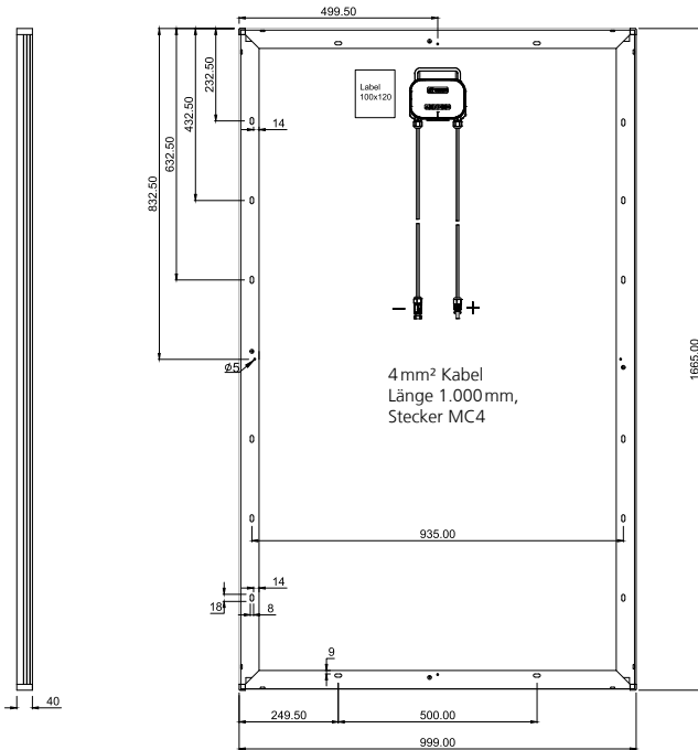
WSP-Serie Rückansicht
